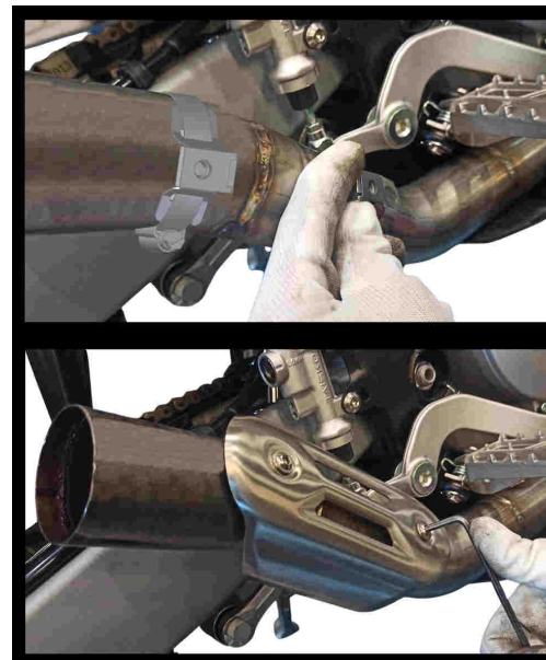
RIMONTAGGIO COVER ORIGINALE ORIGINAL COVER REASSEMBLY
