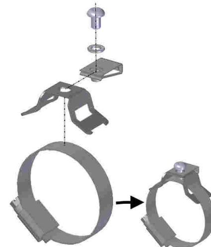
APRIRE LA FASCETTA PER INSERIRE LA STAFFA REGOLABILE OPEN THE CLAMP TO INSERT THE ADJUSTABLE BRACKET
